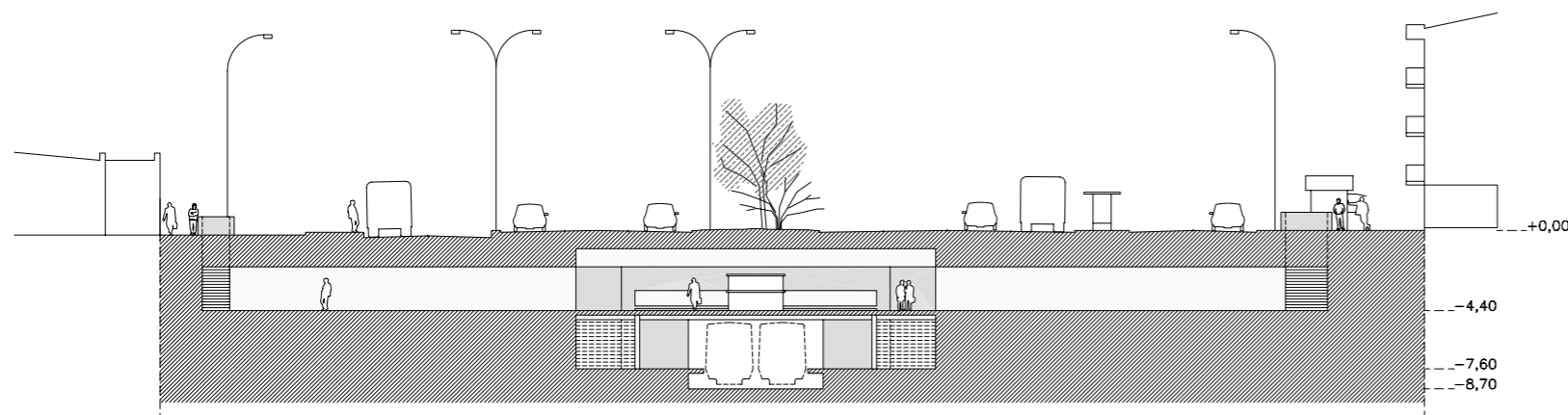
SECCION A-A
