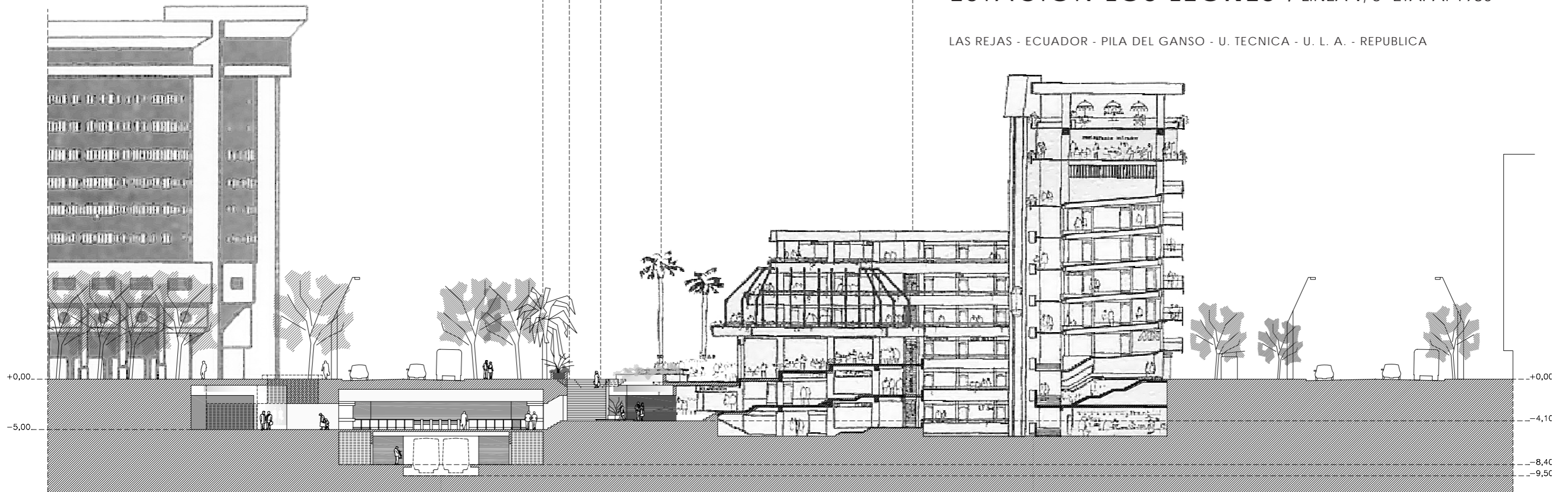
SECCION A-A
