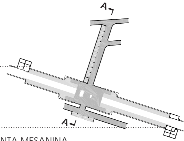
PLANTA MESANINA Y SALIDAS
