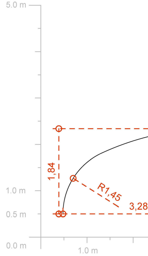
TIPOLOGIA 38 - TRAÇA 27 - GEOMETRIA 16 Redibuixat: CS1.N1
