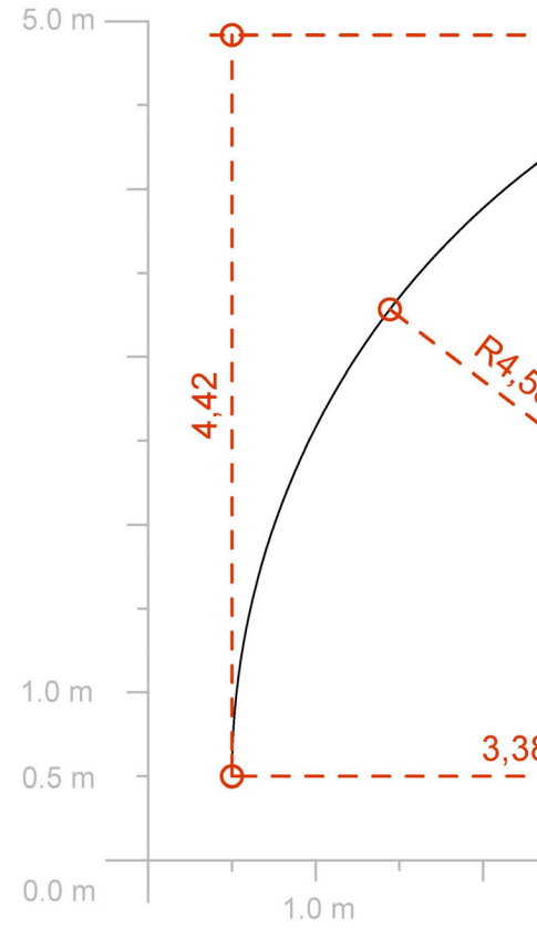
TIPOLOGIA 26 - TRAÇA 17 - GEOMETRIA 11 Redibuixat: G9.N2
