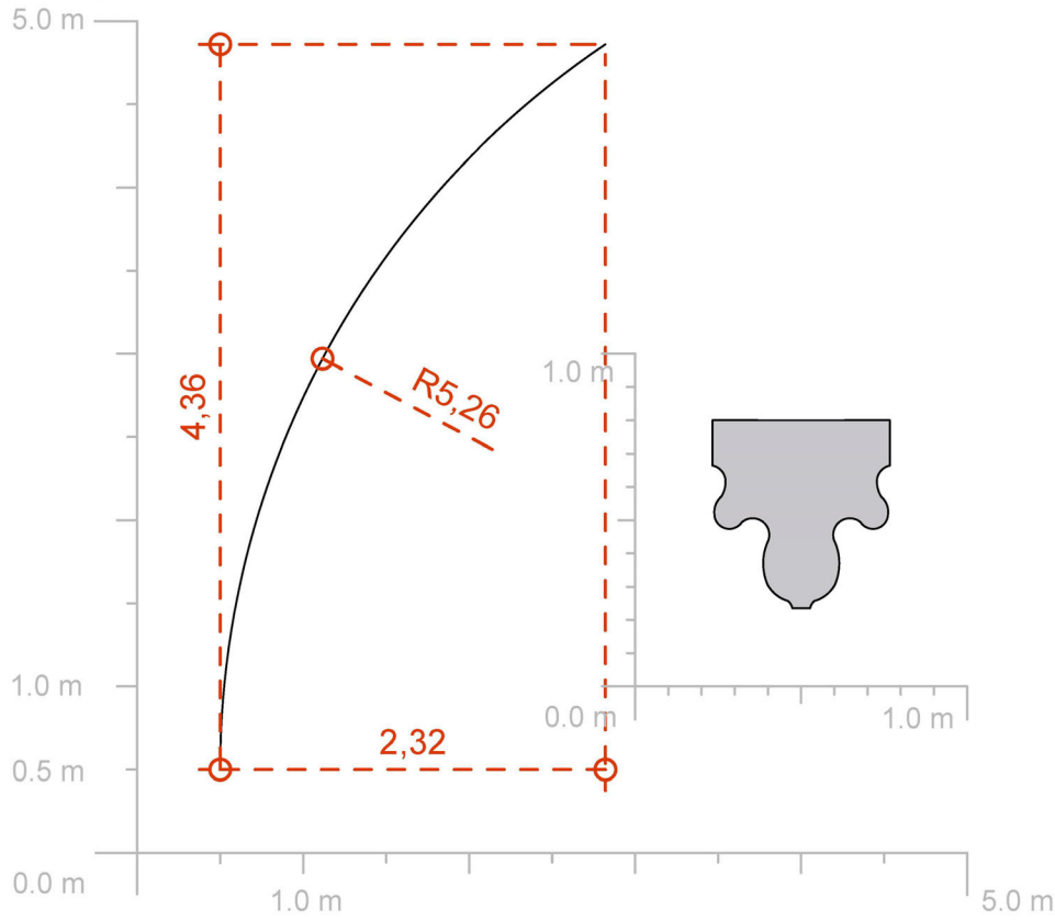
TIPOLOGIA 25 - TRAÇA 16 - GEOMETRIA 10 Redibuixat: A2.5
