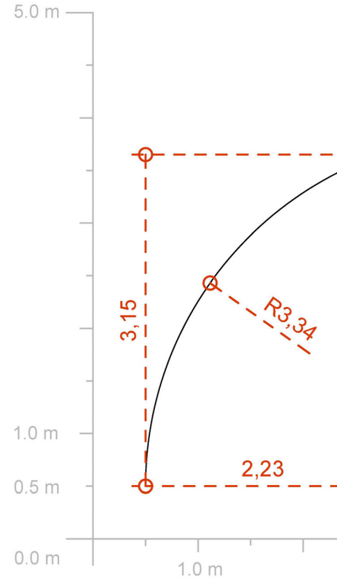
TIPOLOGIA 14 - TRAÇA 9 - GEOMETRIA 1 Redibuixat: A1.30
