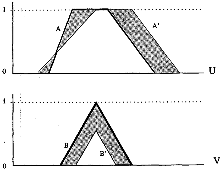
Figura 4.4. L'operador \underline{S}_{AB}^T
