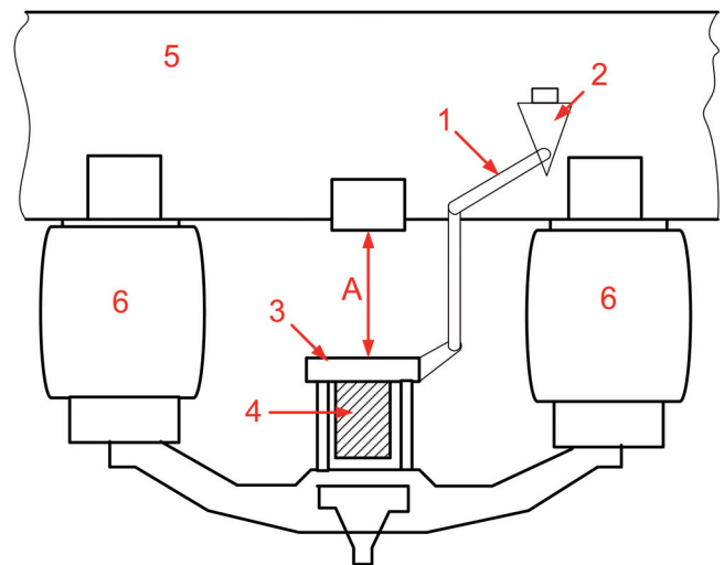
Figura 5: Válvula de Control de Nivel en vehículos con suspensión neumática
