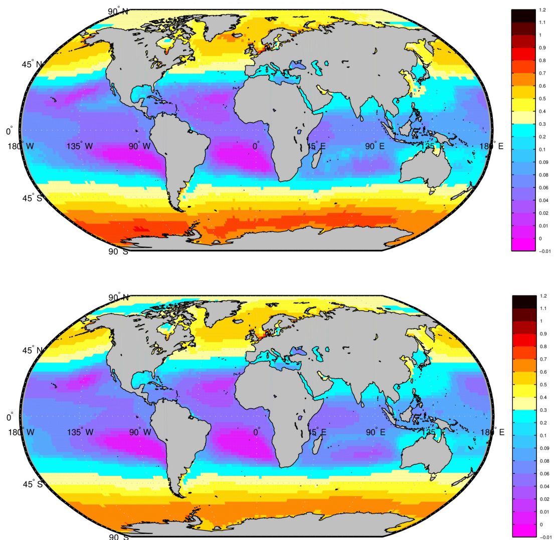
Figura 11: Valor del percentil del 99.5% (m) de la reconstrucción estadística utilizando 20CR para el periodo 1992-2010 (panel superior) y para el periodo completo de 20CR (panel inferior).
