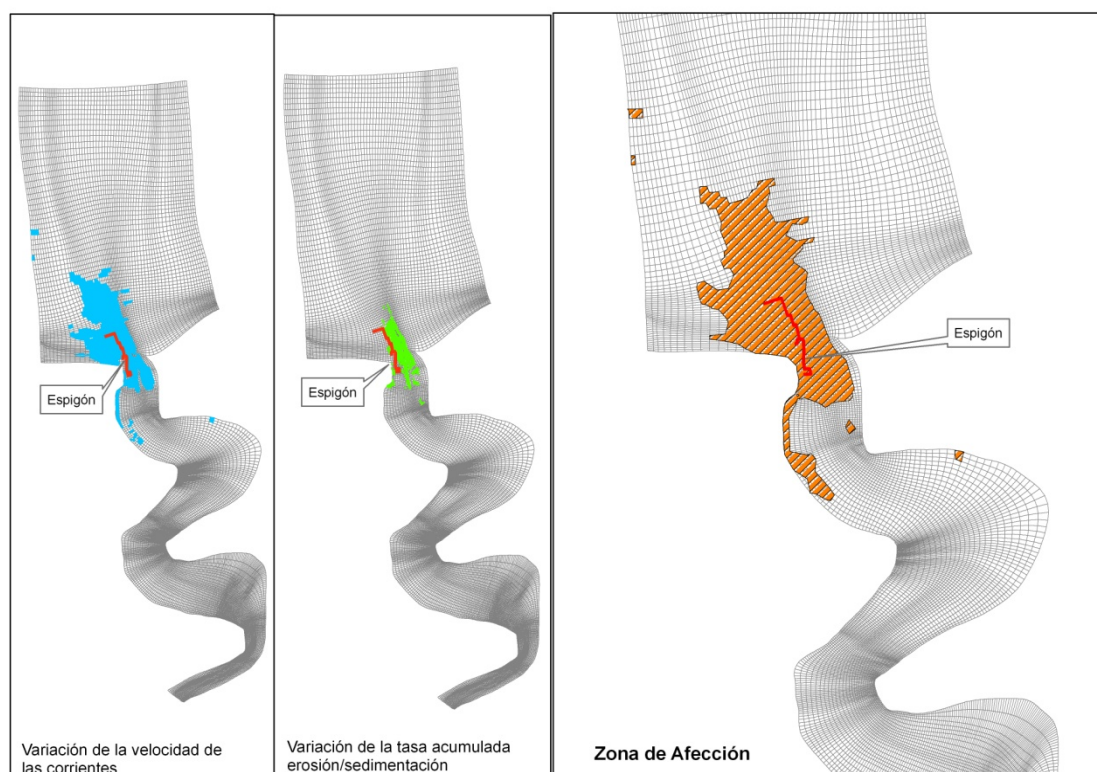
Figura VI. 24. Zona de afección de un espigón teórico situado la bocana de la ría.
