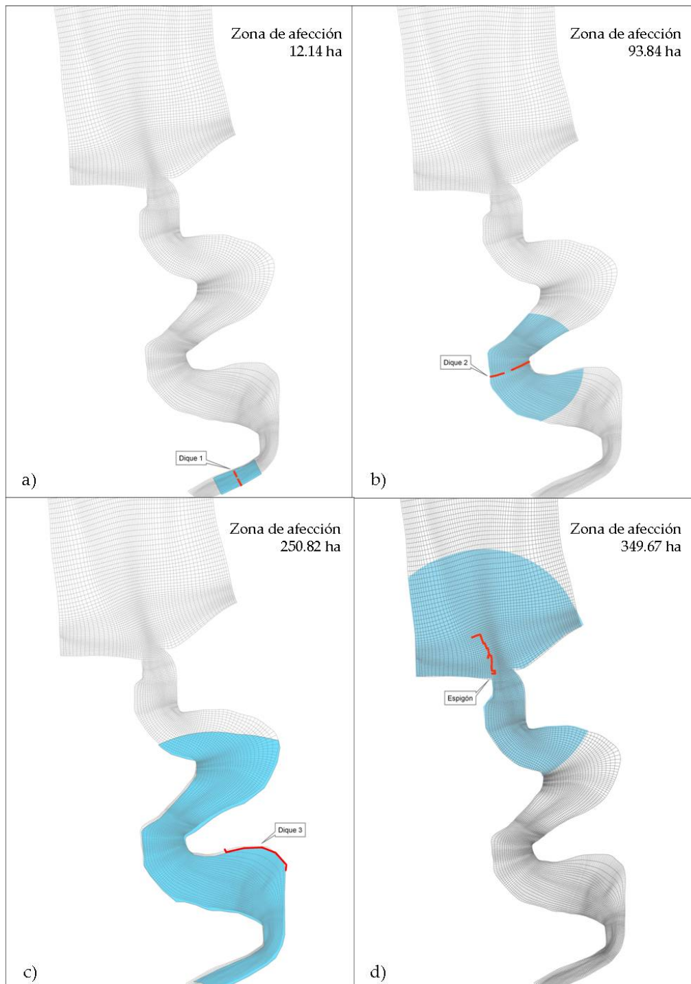
Figura VI. 25. Zona de afección delimitada mediante el método estático para las alteraciones hidromorfológicas teóricas situadas en la Ría de San Martín: a) dique localizado en la cola del estuario; b) dique situado en el tramo medio del estuario; c) dique paralelo a la línea de tierra; y d) espigón situado en la bocana de la Ría.
