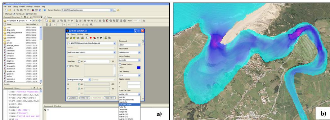
Figura VI. 6. Transformación de los resultados del modelo hidrodinámico: a) exportación de datos a formato ARCview shape y b) ráster generado a partir de los resultados del modelo.
