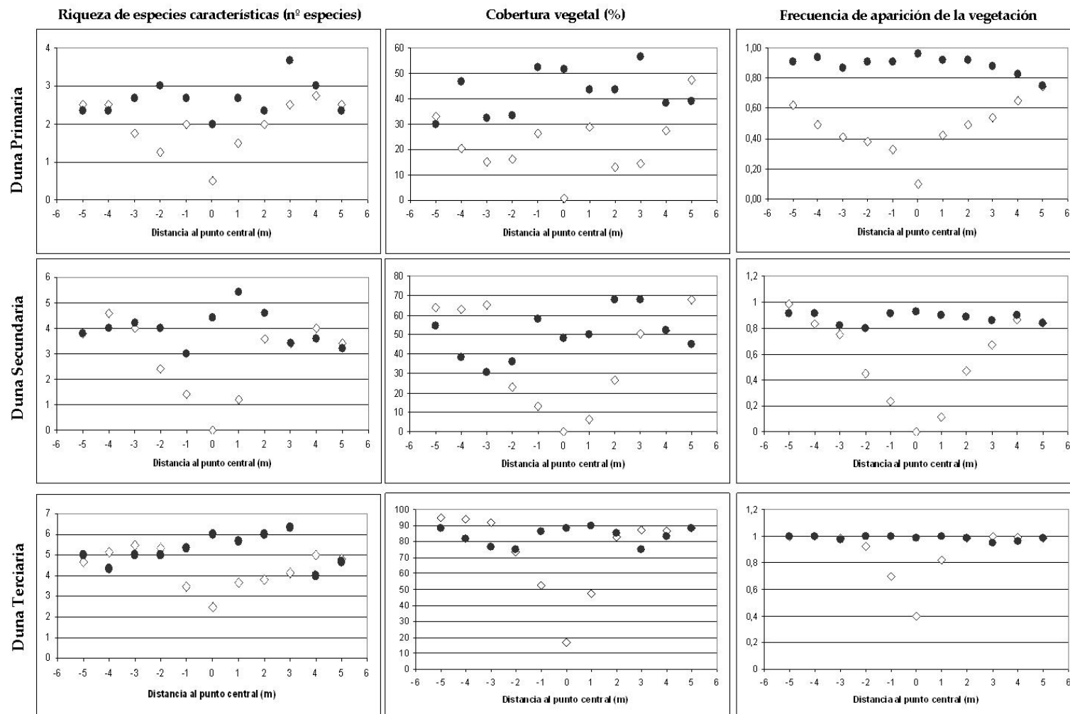
Figura V. 14. Valores medios de la riqueza de especies características, cobertura vegetal (%) y frecuencia de aparición de la vegetación (tanto por 1) en los diferentes estratos dunares (◇= estaciones localizadas en sendas transitadas; ●= estaciones control).
