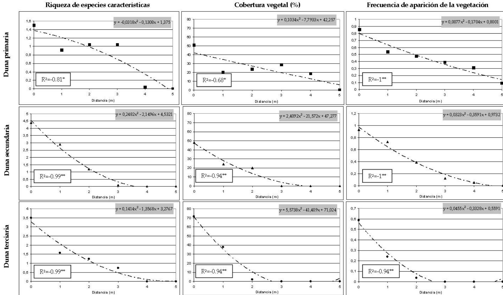
Figura V. 15. Diferencias entre los valores medios en las unidades experimentales control y las sometidas a tránsito, para las cinco distancias al punto central de la senda analizadas: representación gráfica de las líneas de regresión, y coeficientes de correlación de Spearman (R 2 ).
