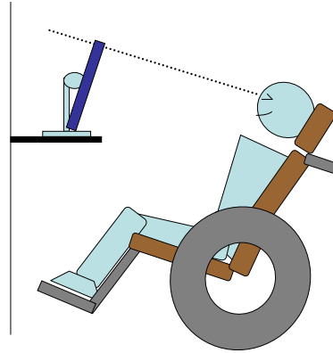
Figura 6. Altura e inclinación de la pantalla para usuarios con postura de referencia reclinada o en apoyo posterior.
