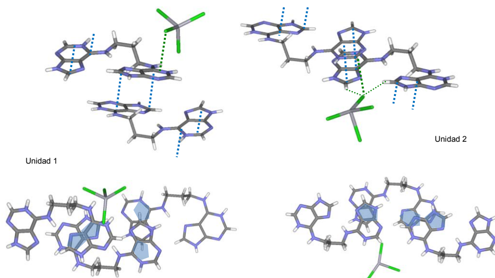
Figura 99. Comparación de las interacciones anión- \pi (verde) y de apilamiento (azul) en las dos unidades de la estructura de N 6 -[(H-Ade) 2 C 3 ] [HgCl 4 ]·3H 2 O (vista lateral y apical).
