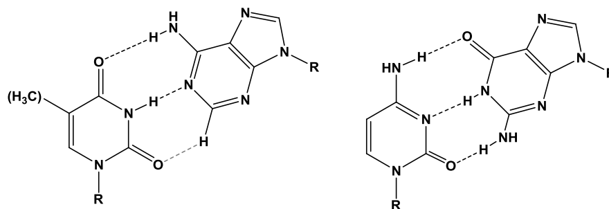
Figura 24. Interacción Adenina-Timina (o Uracilo) y Guanina-Citosina tipo Watson-Crick.
