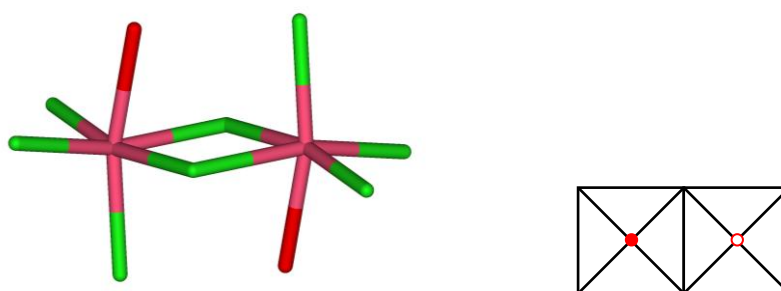
Figura 63. Dímero [Cd_2Cl_8(H_2O)_2]^{4-} con N^9-Ade_2C_3 . Al lado, representación esquemática del anión de Cd(II) (cada unidad se representa por un octaedro visto desde la posición apical) 70
