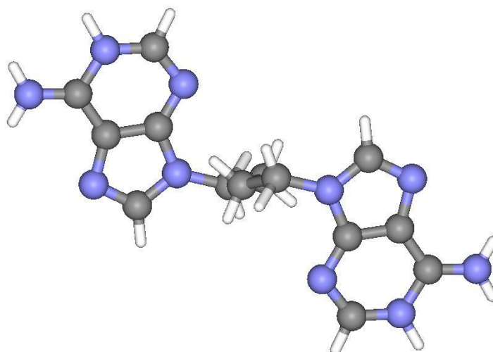
Figura 62. Conformación del ligando en \{N^9-[(H-Ade)_2C_4]_2 [Cd_4Cl_{12}(H_2O)_2] \cdot 4 H_2O\}_\infty
