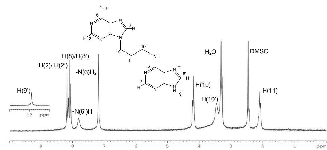
Figura 108. Espectro de ^1\text{H} -RMN de \text{N}^{9,6'} - \text{Ade}_2\text{C}_3
