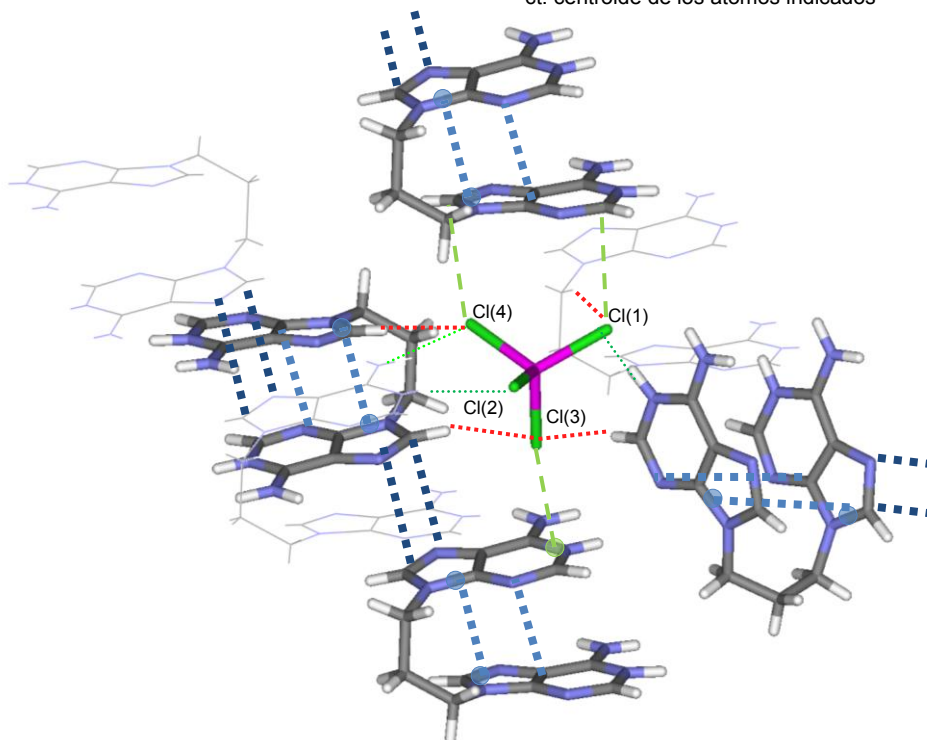
Figura 60. Interacciones intermoleculares débiles en N 9 -[(H-Ade) 2 C 3 ] [ZnCl 4 ] · H 2 O ( stacking marcado en azul, las interacciones tipo C-H···Cl marcadas en rojo y las anión- \pi marcadas en verde).
