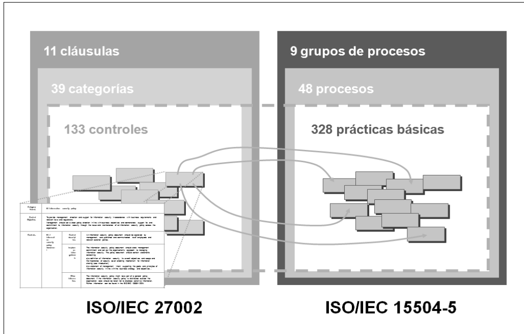
Figura 4.2. Procedimiento seguido para el estudio de las relaciones entre las normas ISO/IEC 27002 e ISO/IEC 15504-5
