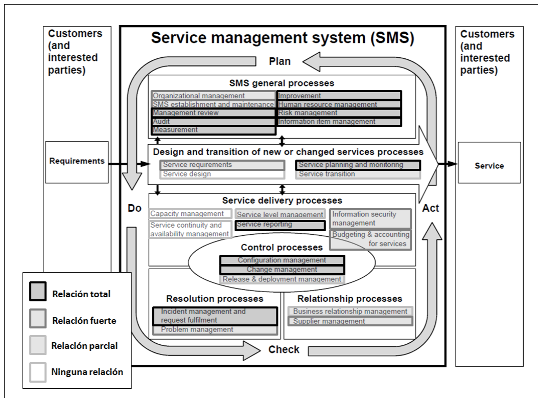
Figura 3.5. Grado de cobertura de los procesos de ISO/IEC 20000-4 por la norma ISO/IEC 15504-5
