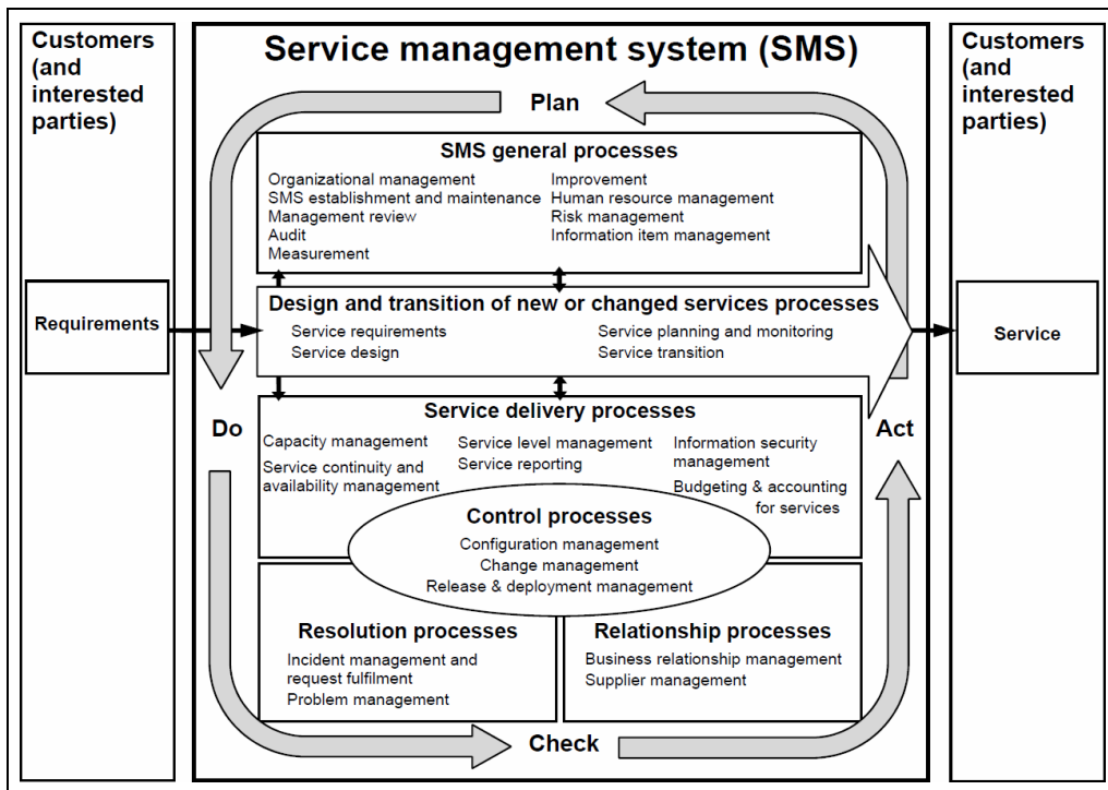
Figura 2.5. Sistema de gestión de servicios de TI de la norma ISO/IEC 20000
