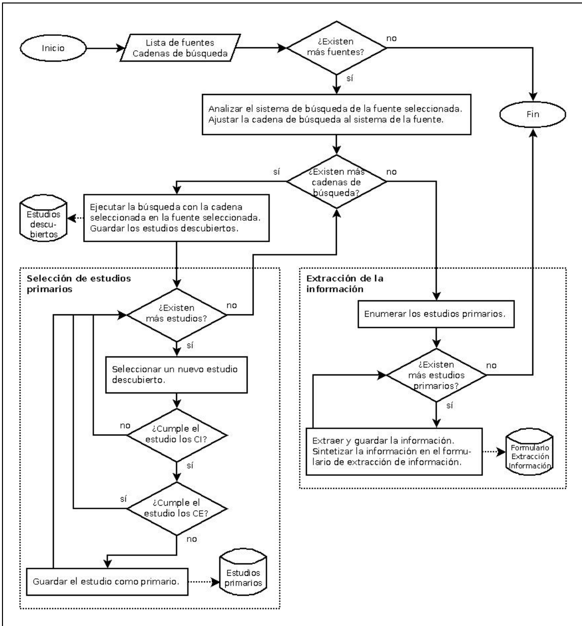
Figura A.1. Procedimiento para la ejecución de la revisión sistemática
