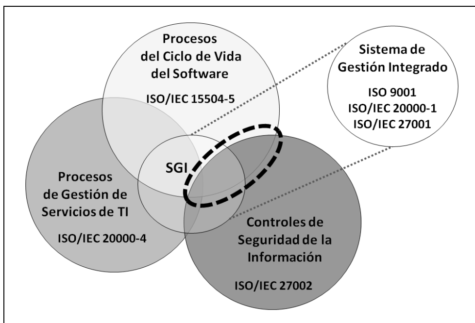
Figura 4.1. Fase II de la construcción del Modelo Integrado de Estándares de Gestión de TI
