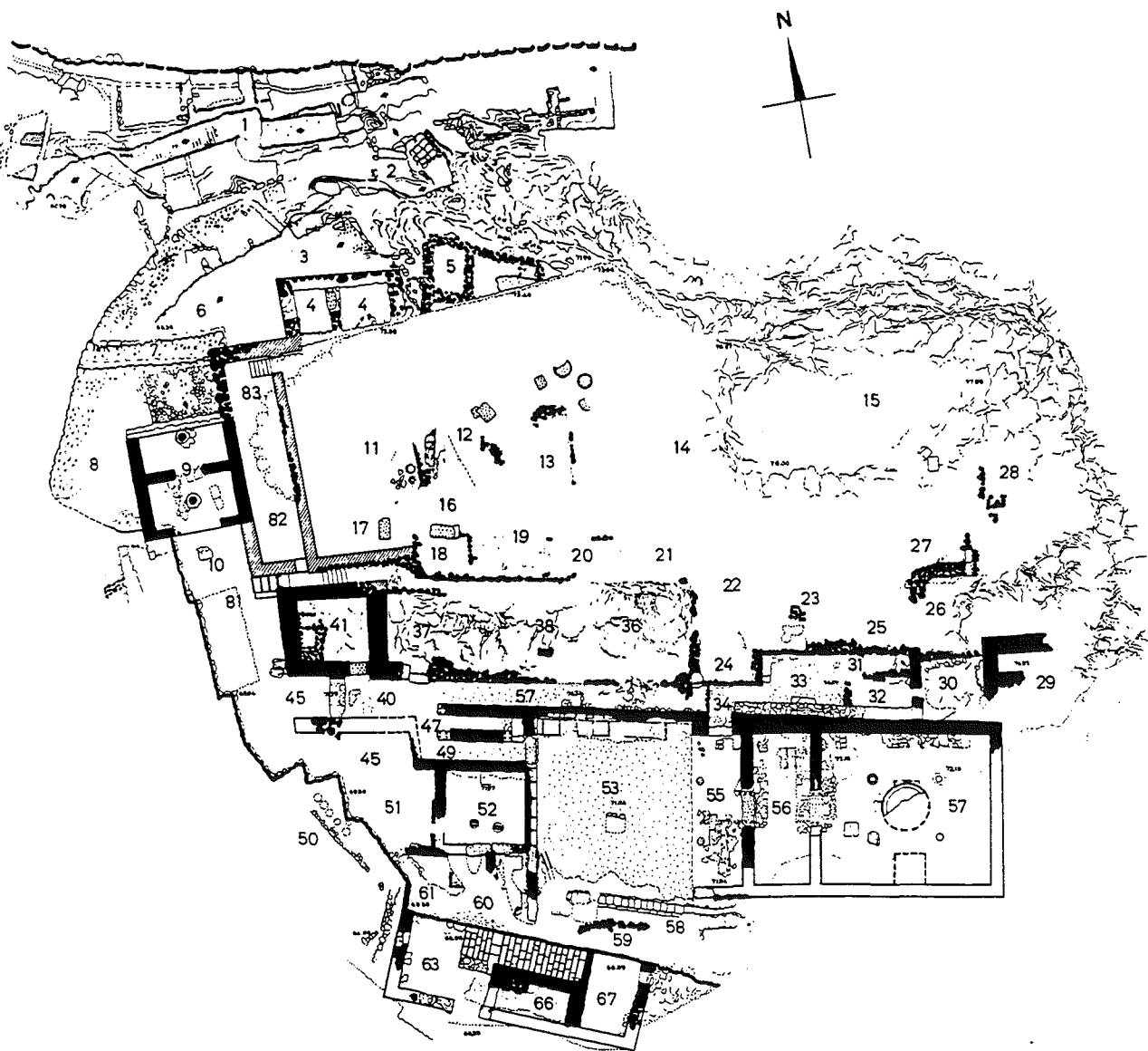
Plano XVI: Palacio de Micenas. Ala principal.
