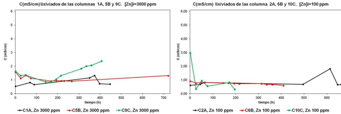
Figura 5. 14. Representación gráfica de la conductividad de los lixiviados frente al tiempo, de las disoluciones de Zn.
