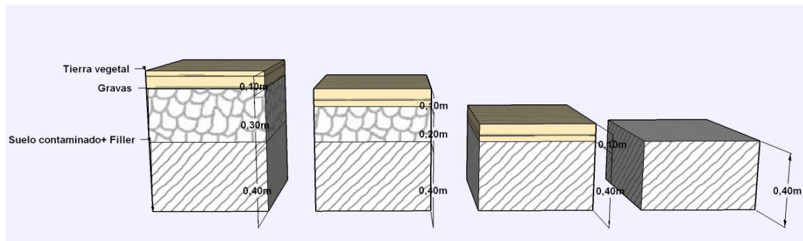
Figura 4. 4. Esquema de las distintas configuraciones de los Tecnosoles, donde varía el porcentaje de la mezcla sedimento-filler y el tipo de cubierta.
