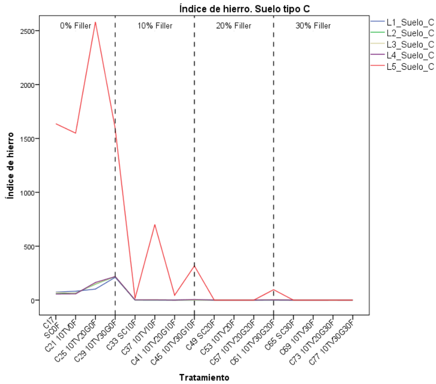
Figura 4. 34. Índice de hierro de los lixiviados del sedimento C.
