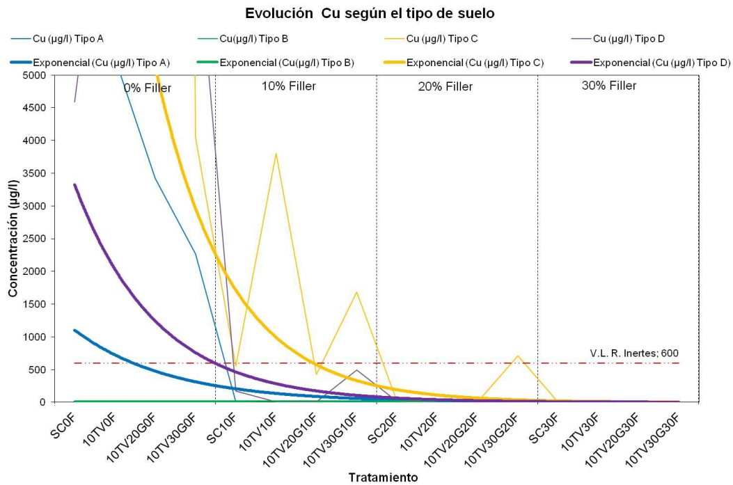
Figura 4. 23. Detalle de la regresión exponencial de los datos del cobre.
