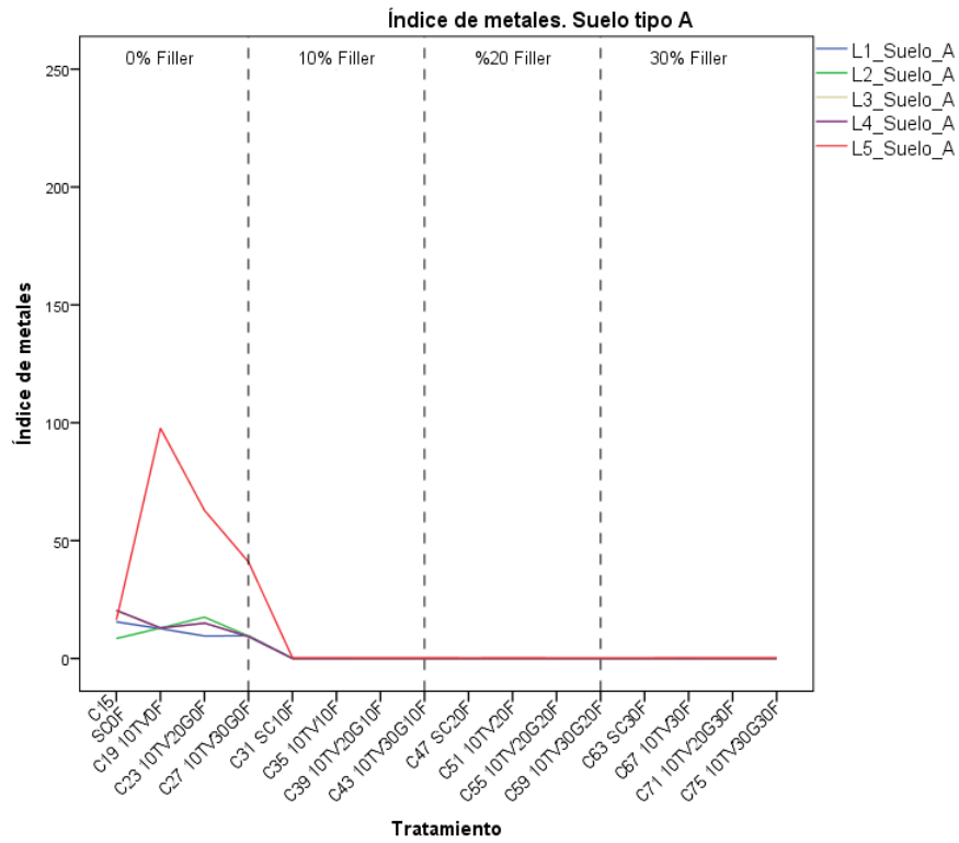
Figura 4. 28. Índice de EPTs de los lixiviados del sedimento A.
