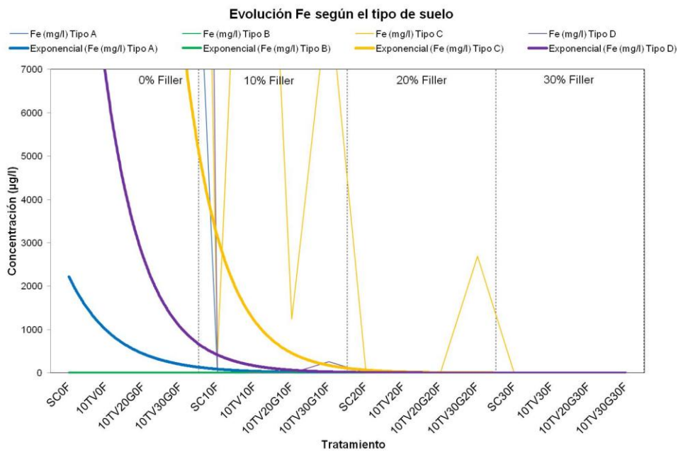
Figura 4. 17. Detalle de la regresión exponencial de los datos del hierro.
