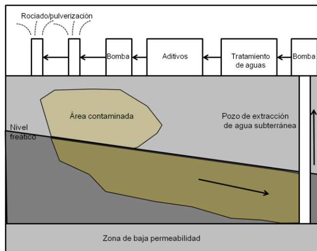
Figura 1. 6. Esquema del enjuague in situ (FRTR, 2002).
