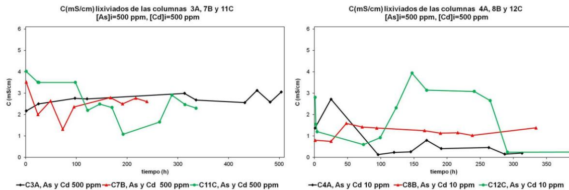
Figura 5. 15. Representación gráfica de la conductividad de los lixiviados frente al tiempo, de las disoluciones As y Cd.
