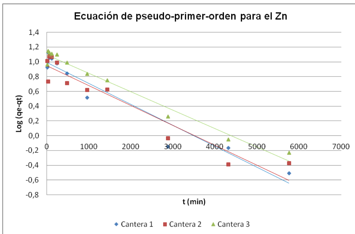
Figura 3. 16. Gráfico \log (q_e - q_t) frente a t para el cinc.
