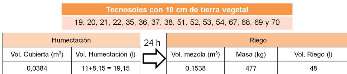
Figura 4. 10. Volumen de riego total de los Tecnosoles con 10 cm de tierra vegetal.
