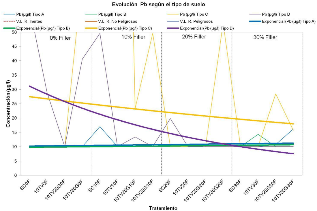
Figura 4. 25. Detalle de la regresión exponencial de los datos del plomo.
