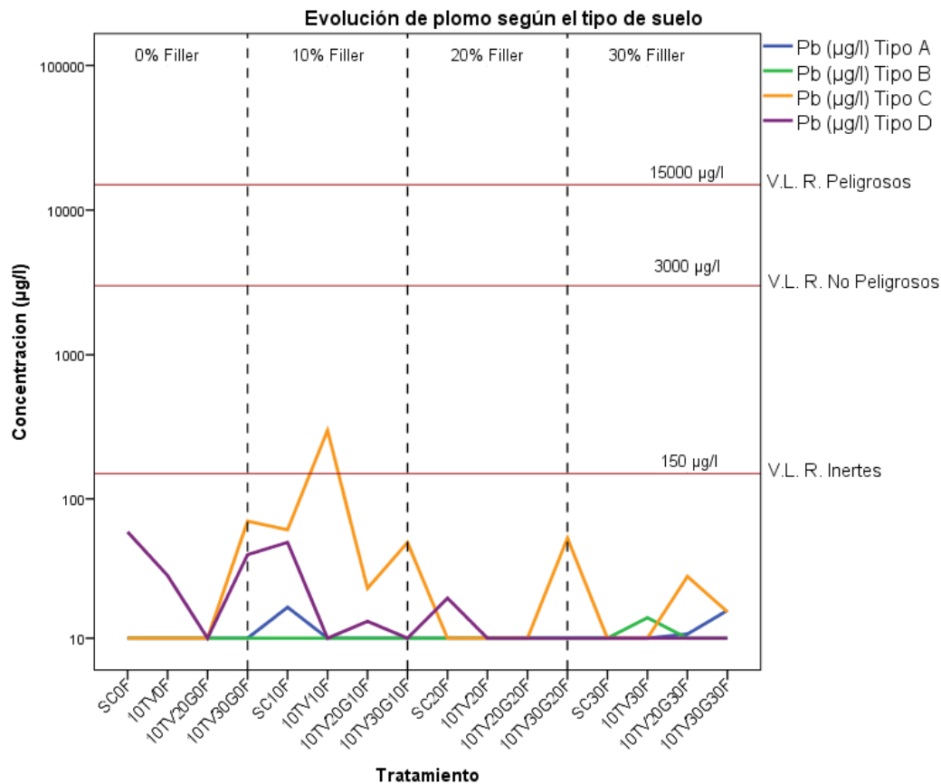
Figura 4. 24. Evolución del plomo en función del tratamiento en el riego.
