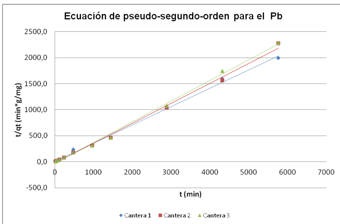
Figura 3. 21. Gráfico t/q_t frente a t para el plomo.
