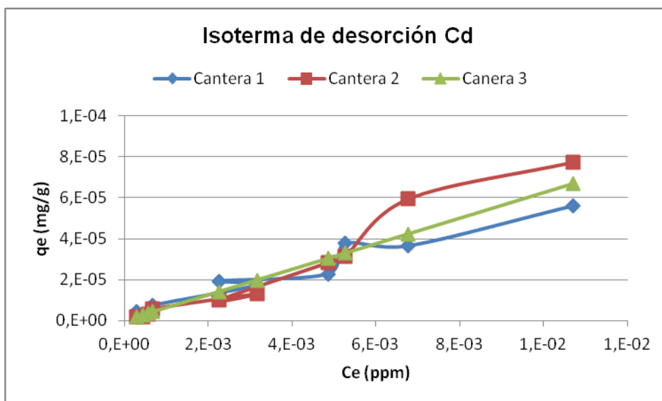
Figura 3. 23. Isoterma de desorción del cadmio.
