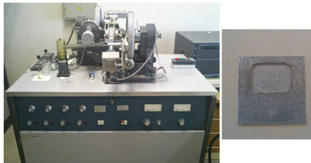
Figura A. 2. Equipo de Difracción de Rayos X (DRX) y porta muestras.
