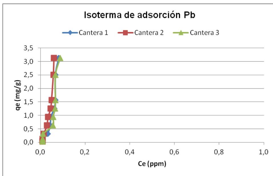
Figura 3. 9. Isoterma de adsorción del plomo.
