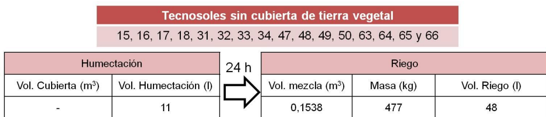
Figura 4. 9. Volumen de riego total de los suelos sin cubierta.
