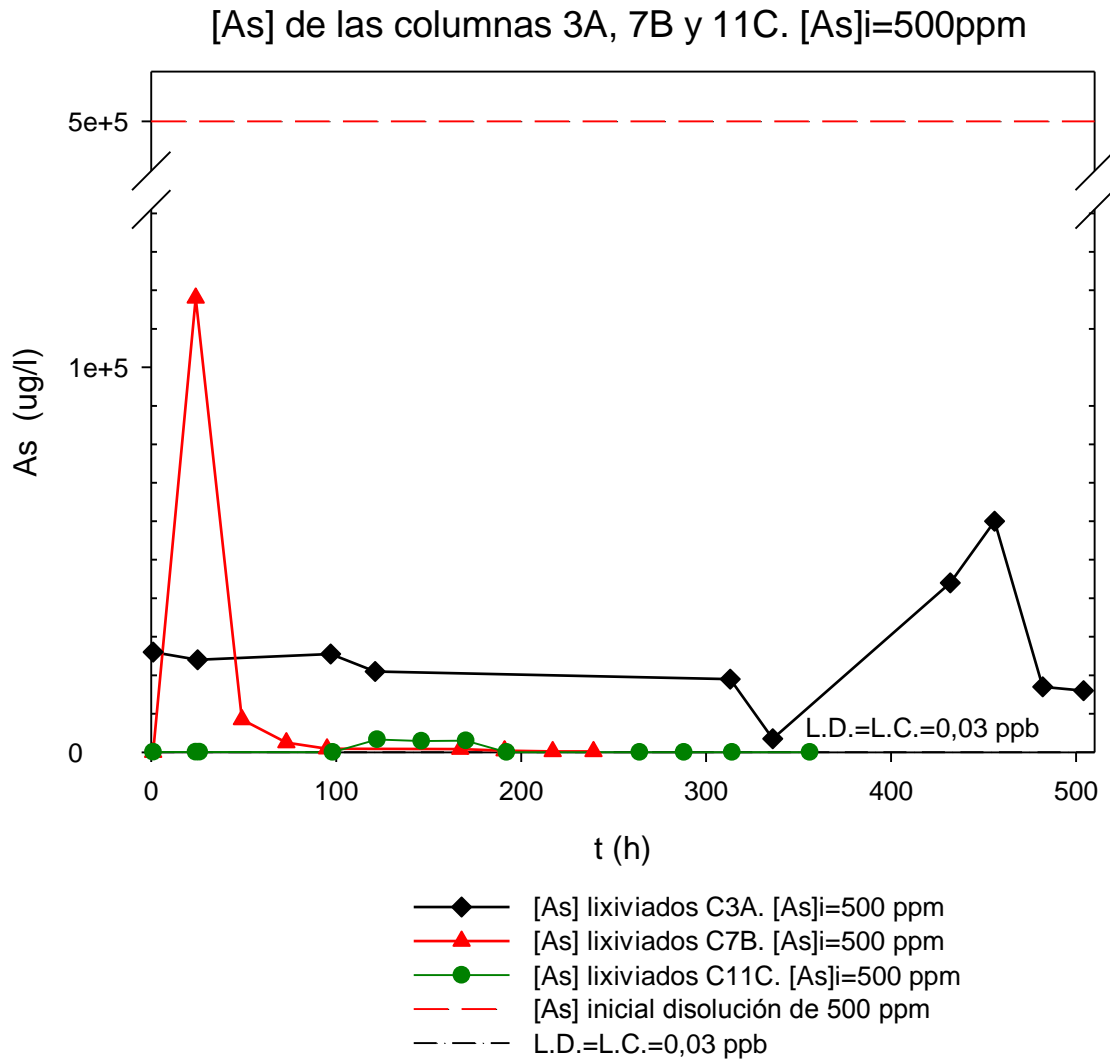
Figura 5. 20. Concentración de As de los lixiviados en las columnas 3A, 7B y 11C frente al tiempo, para una disolución inicial de As de 500 ppm.
