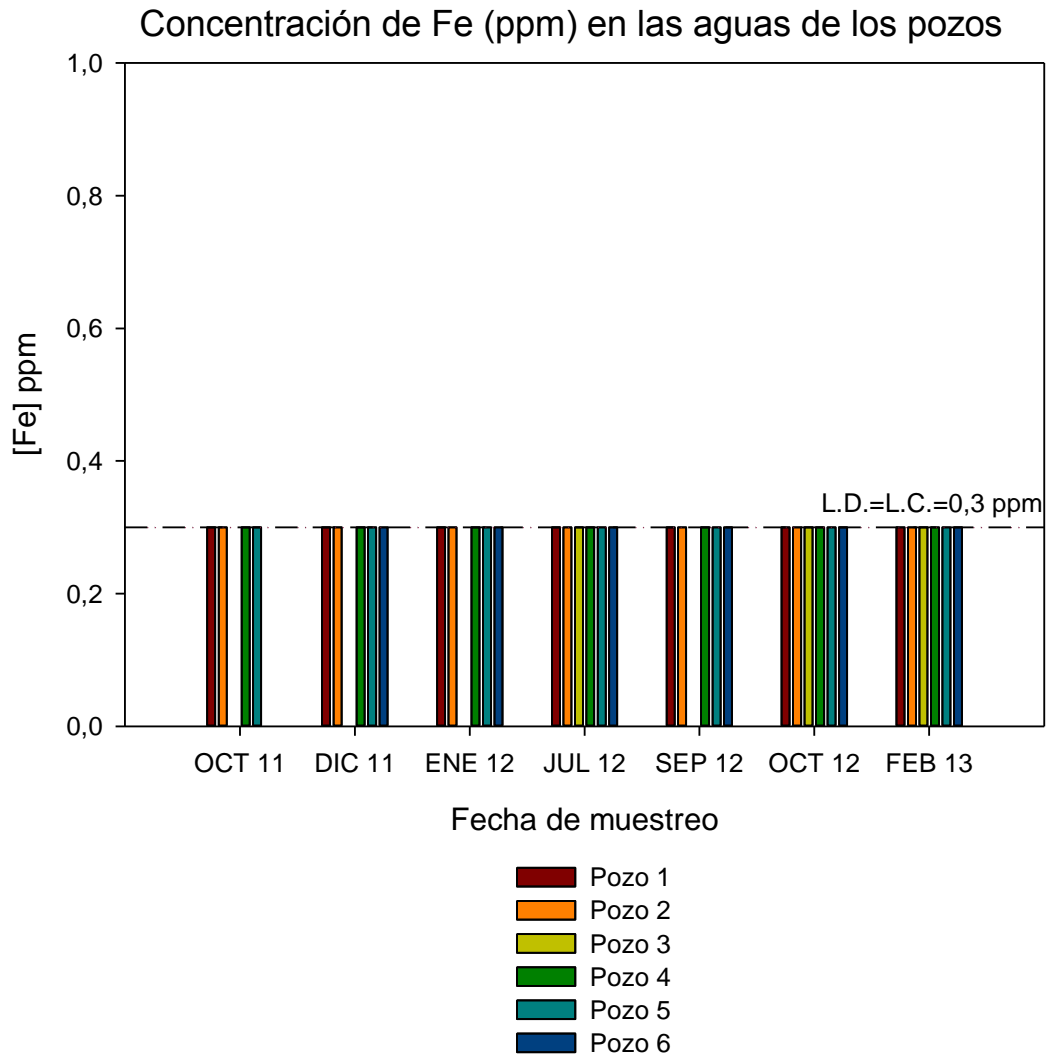
Figura 5. 28. Concentración de hierro en las aguas de los pozos de las barreras, frente a la fecha de muestreo.
