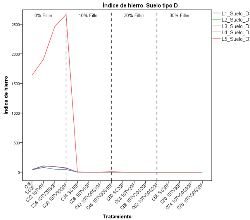
Figura 4. 35. Índice de hierro de los lixiviados del sedimento D.
