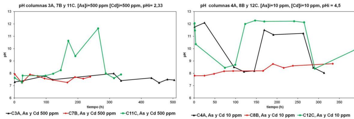
Figura 5. 12. Representación gráfica del pH de los lixiviados frente al tiempo, de las disoluciones As y Cd.
