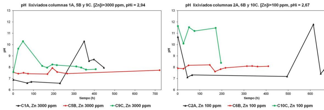
Figura 5. 11. Representación gráfica del pH de los lixiviados frente al tiempo, de las disoluciones de Zn.
