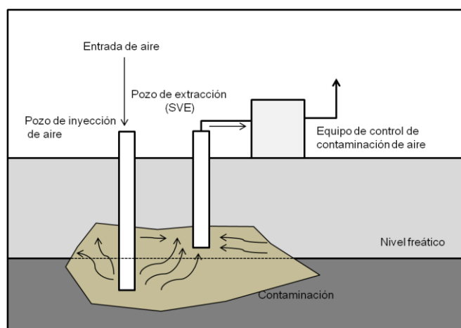
Figura 1. 5. Esquema de la Extracción de vapores de suelo y aspersión de aire (US EPA, 2001a).
