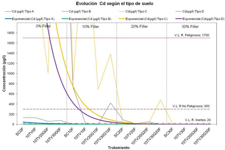
Figura 4. 21. Detalle de la regresión exponencial de los datos del cadmio.
