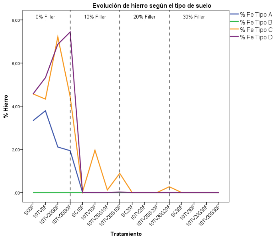
Figura 4. 16. Evolución del hierro en función del tratamiento en el riego.
