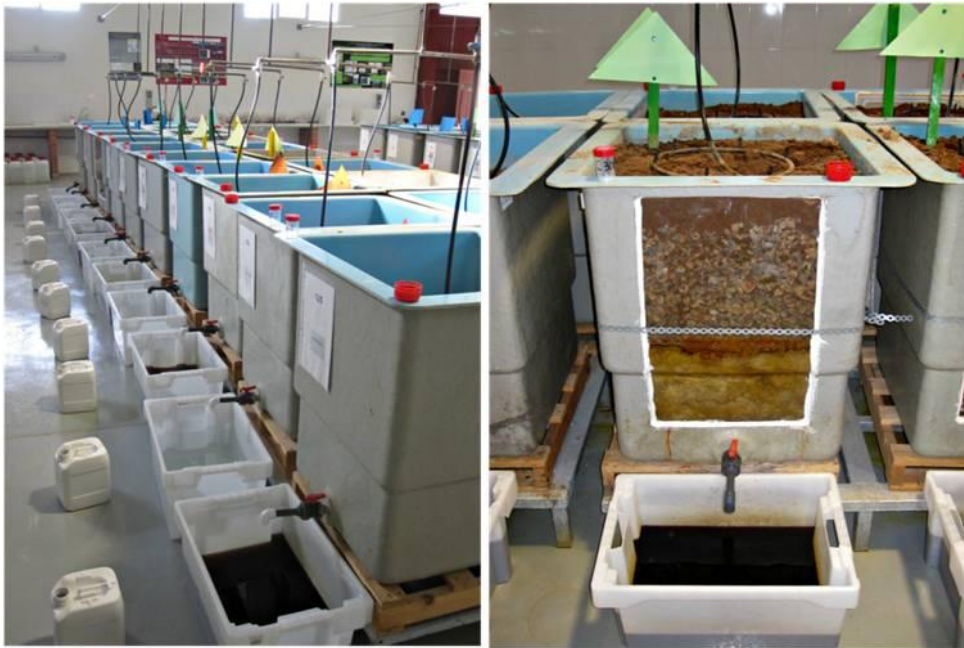
Figura 4. 13. Recogida de lixiviados.
