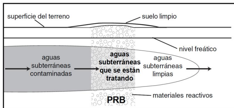
Figura 1. 11. Esquema de una barrera reactiva permeable (US EPA, 2001c).
