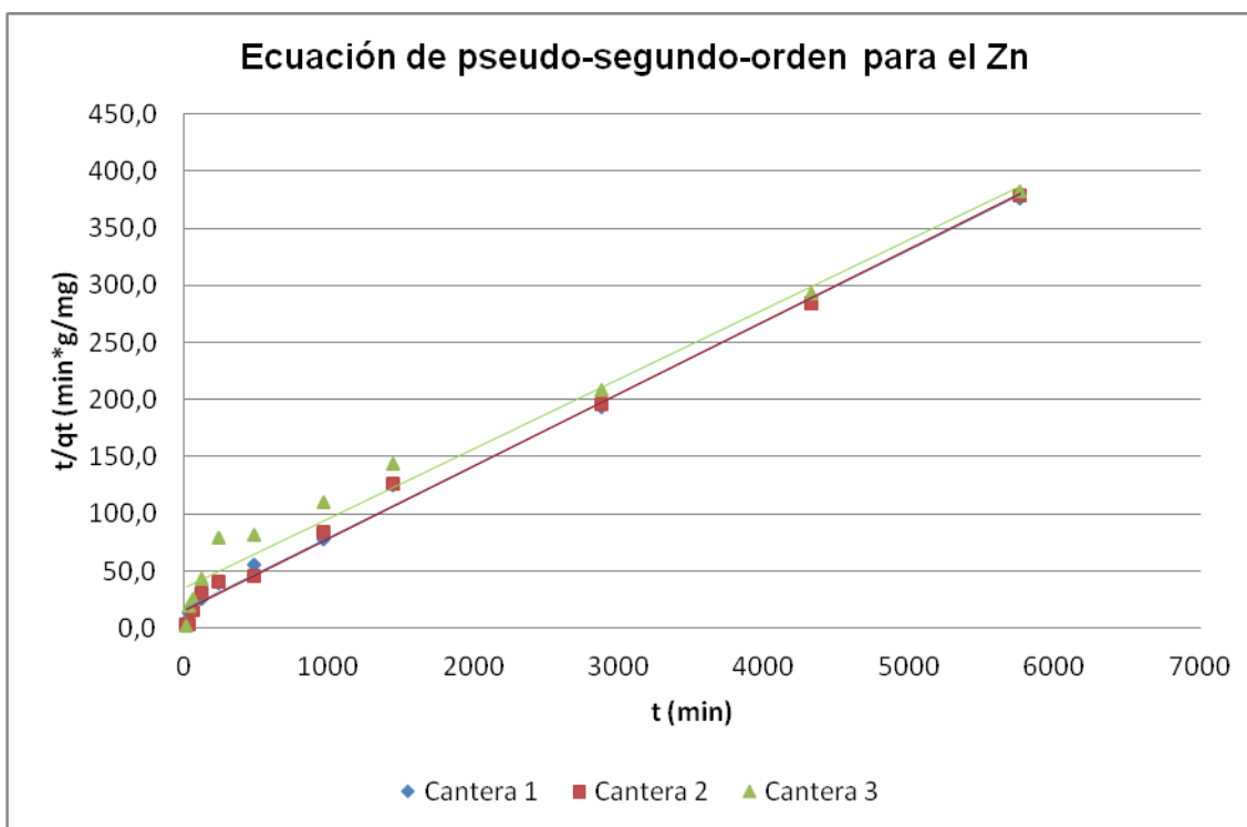
Figura 3. 19. Gráfico t/q_t frente a t para el cinc.
