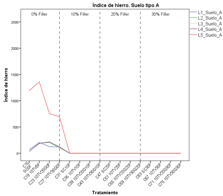
Figura 4. 32. Índice de hierro de los lixiviados del sedimento A.
