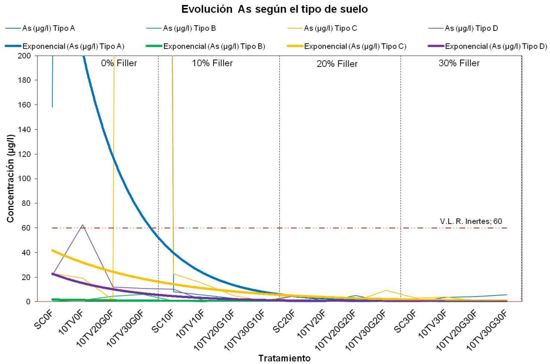
Figura 4. 19. Detalle de la regresión exponencial de los datos del arsénico.
