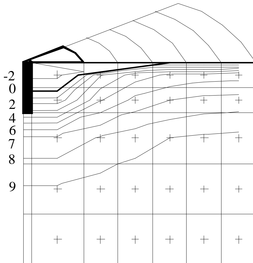
Fig. 29. Resultados del modelo de migración con captación, P_{\text{pozo}} = -10 mmca
