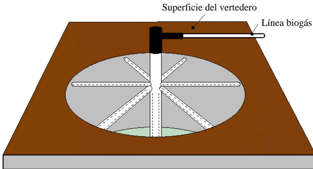
Fig. 37. Captación radial de biogás
